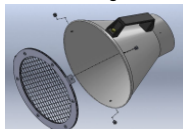
A - Stahl-Kegelhaube
