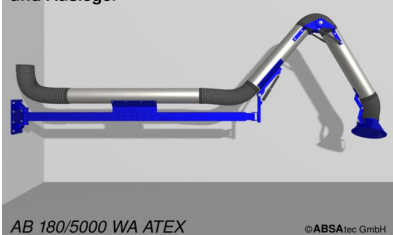
ATEX Absaugarm mit Wandhalterung und Kegelhaube und Ausleger
